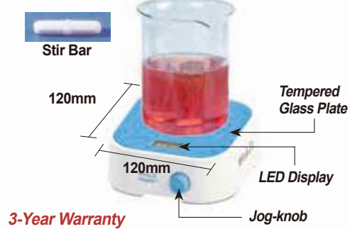
120×120mm Mini Magnetic Stirrer “MS-12D”
