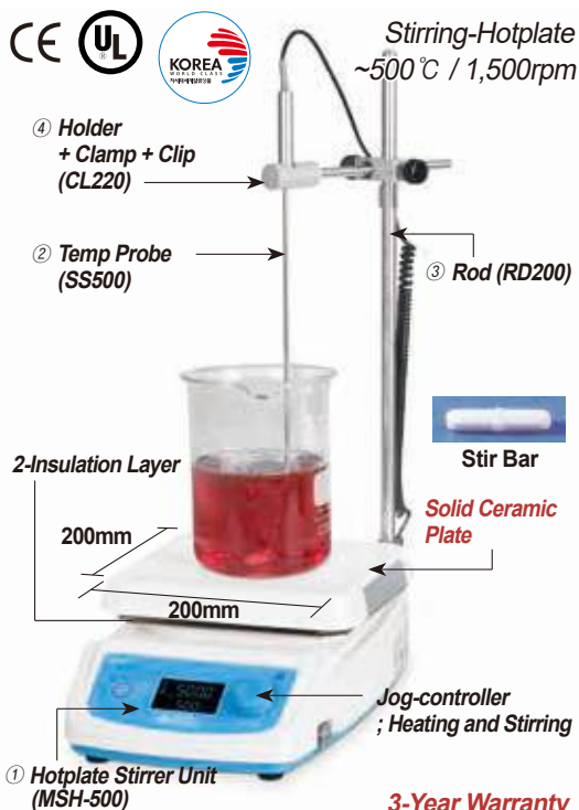
A. “MSH500S” Package-set
